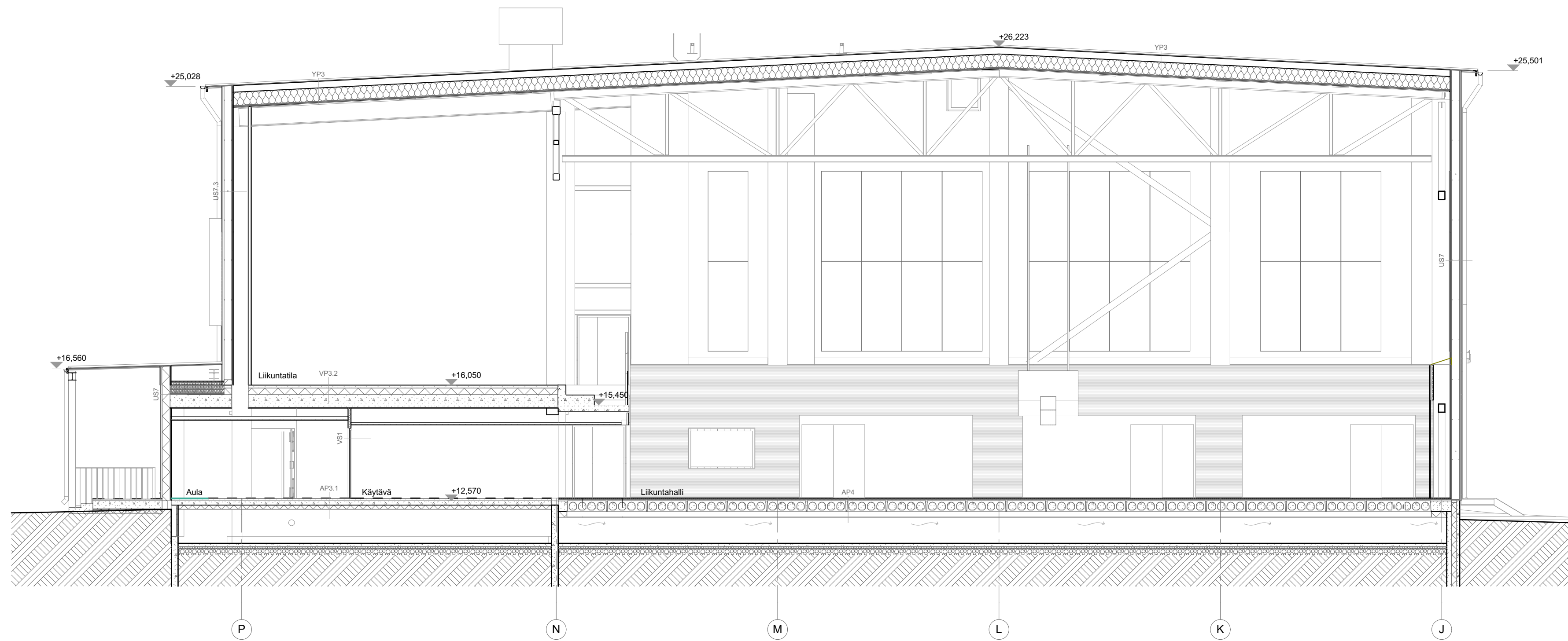
LEIKKAUS A-A, liikuntahalli 1:100
