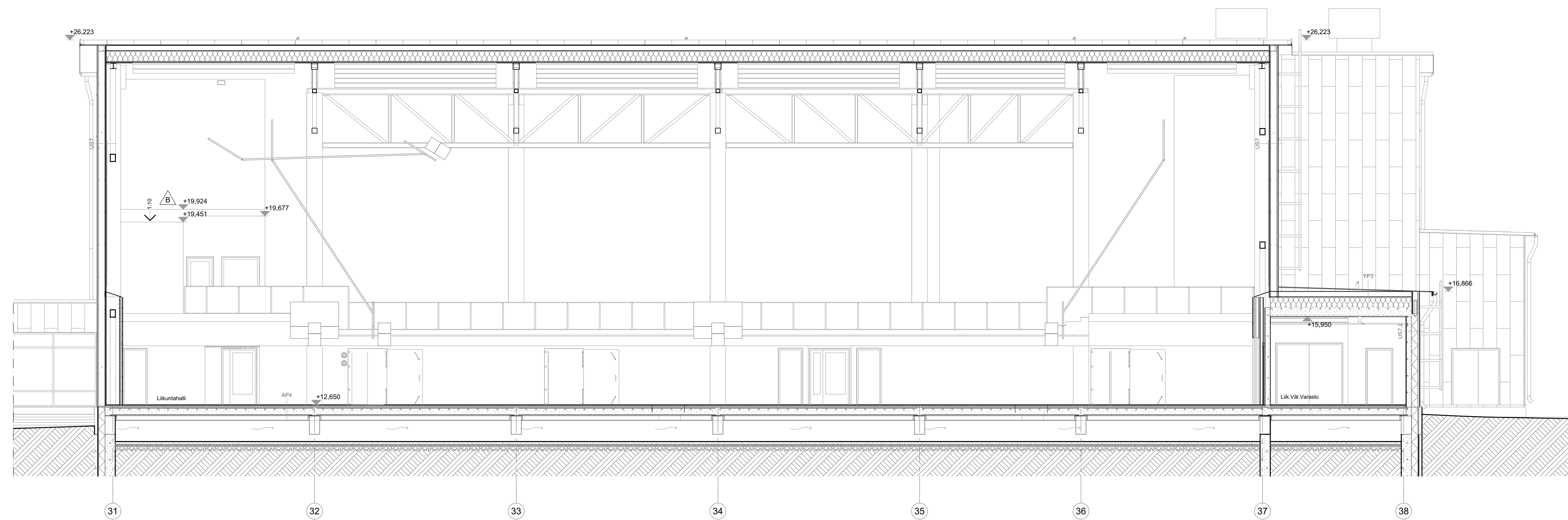
LEIKKAUS B-B, liikuntahalli 1:100
